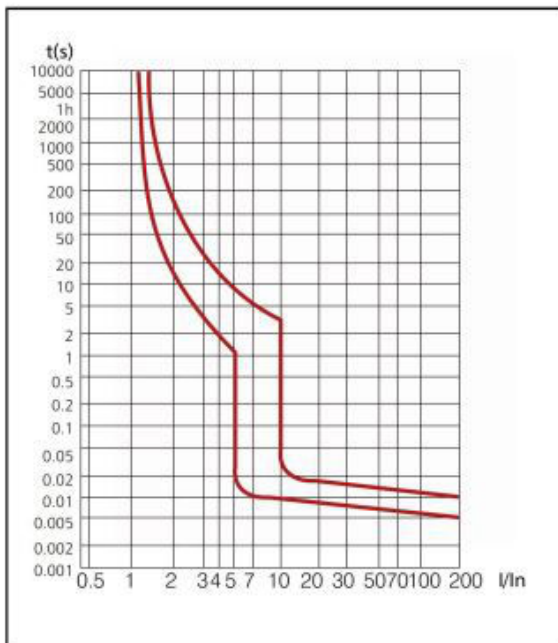
Kennlinie C
