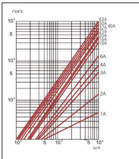
Durchlassenergie I^2t
