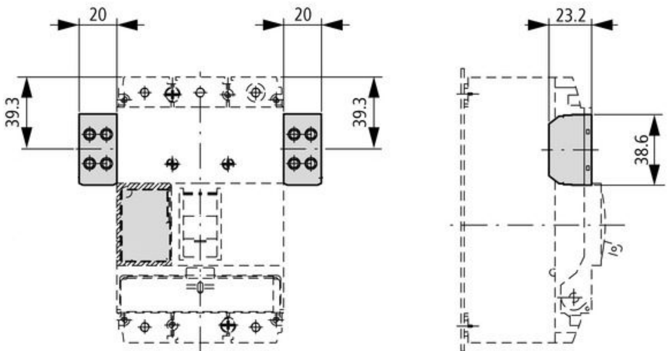
Maßbild: Arbeitsstromauslöser 230VAC/DC + 1 Hiko und 3m Kabel zu MC1
